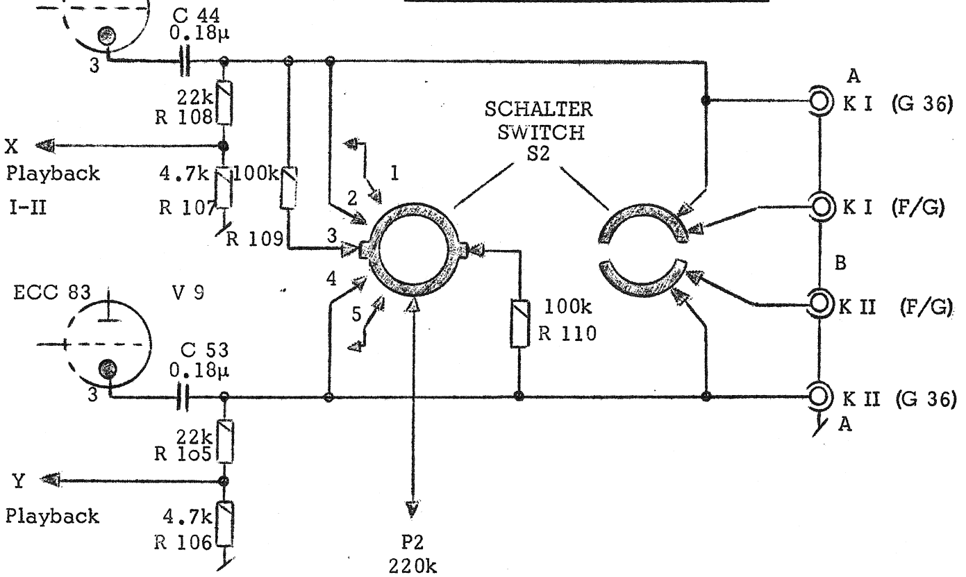
Fig. 2. Kanalwahlschalter S2
