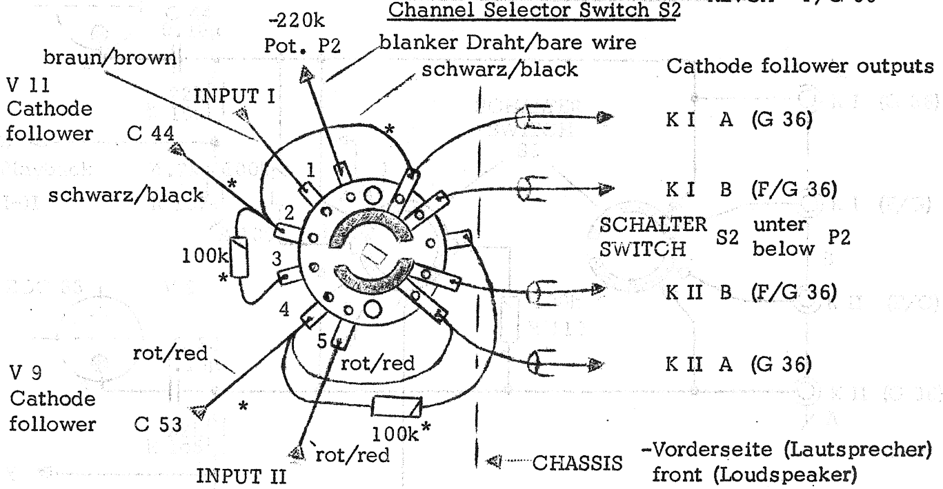
Fig. 2. Kanalwahlschalter S2
